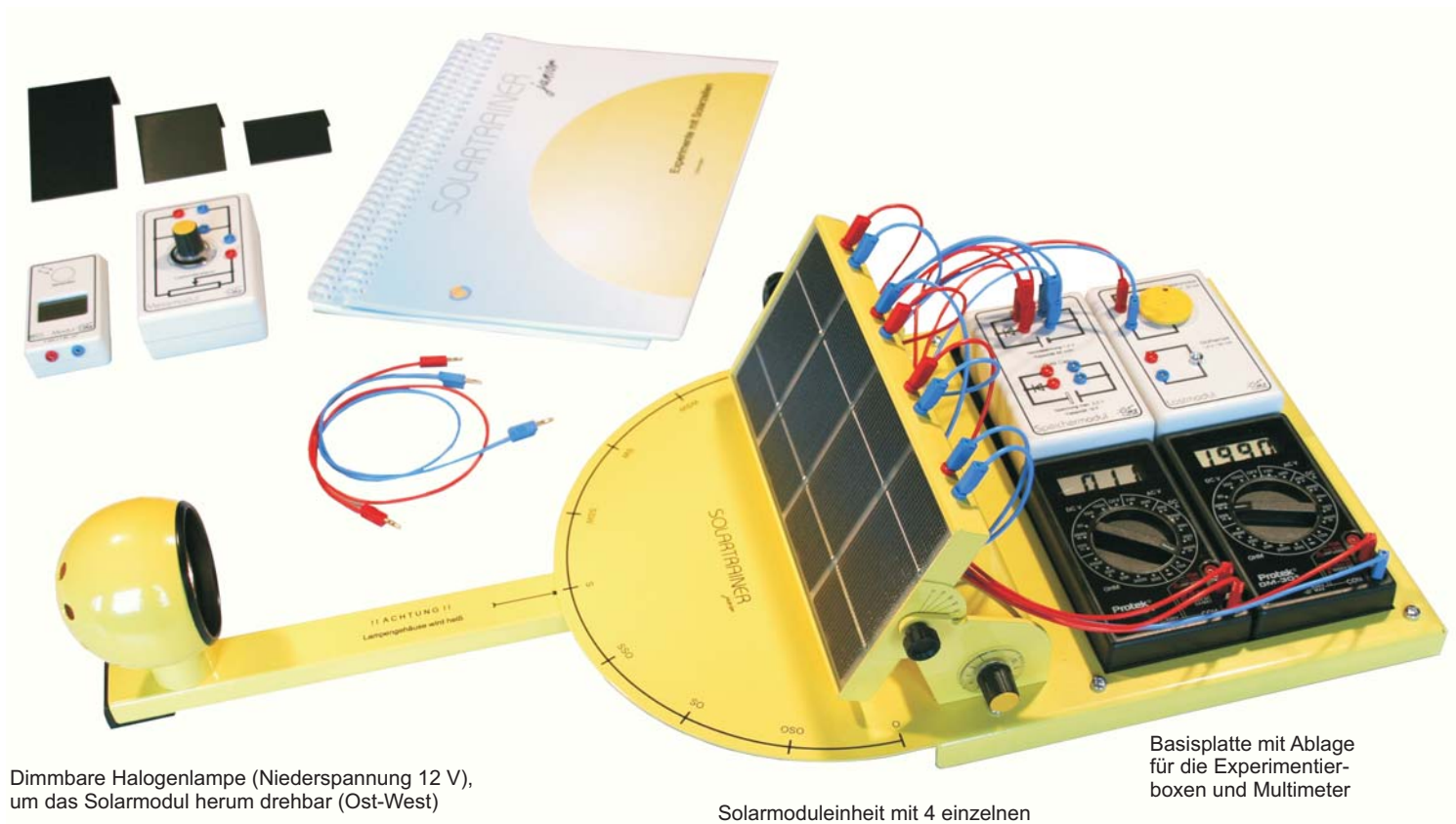
Solarmoduleinheit mit 4 einzelnen Solarzellen, Winkeleinstellung und integrierter Stromversorgung
